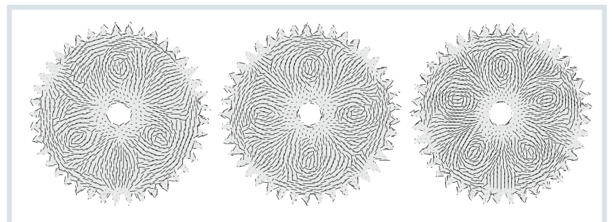
Bild 5. Faserverteilung im Schnitt bei drei, vier und fünf Angüssen. Daraus resultieren unterschiedliche Grade an Schwindung und Verzug © MS-Schramberg
