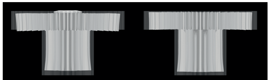
Bild 4. Verformung des Kundenmodells gegenüber der optimierten Geometrie mit Skalierung 5:1. Die größte Verbesserung zeigte das Modell mit den meisten Rippen © MS-Schramberg
