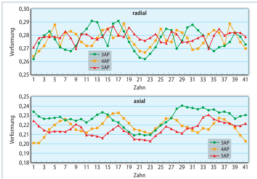
Bild 6. Visualisierung der radialen und axialen Verformung pro Zahn am großen Zahnrad mit drei bis fünf Angüssen (AP = Angusspunkt) Quelle: MS-Schramberg; Grafik: © Hanser
