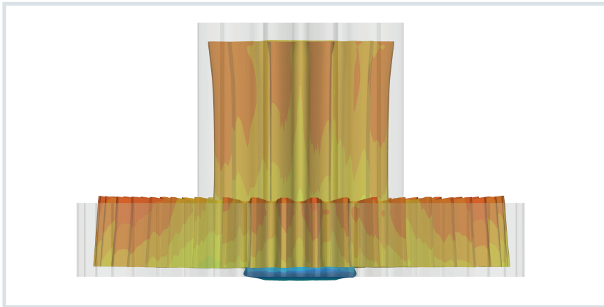
Bild 1. Die erwartete Deformation axial und radial erfordert eine umsichtige Bauteilauslegung (verwendete Skalierung 5:1) © MS-Schramberg
