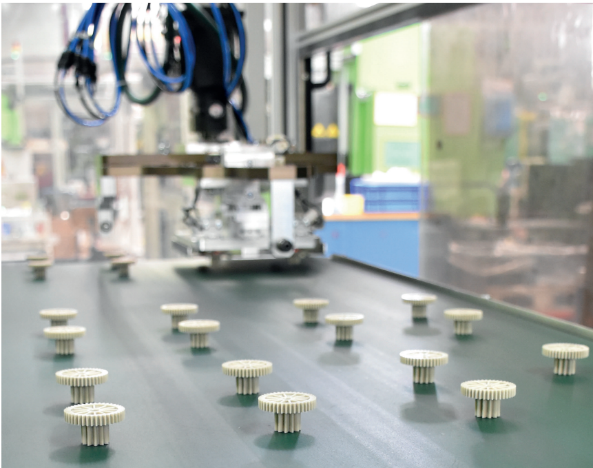
Nach der Bauteiloptimierung lag das Zahnrad in der Serienfertigung von Anfang an innerhalb der gewünschten Toleranz © MS-Schramberg
