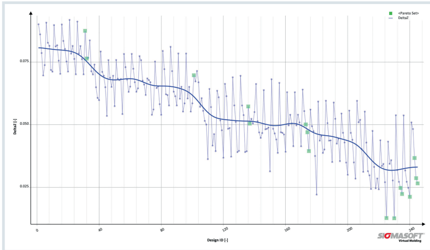
Bild 3. Die Grafik zeigt das Delta Z der 245 Varianten über der Versuchsnummer (nach rechts ansteigende Rippenanzahl) © MS-Schramberg
